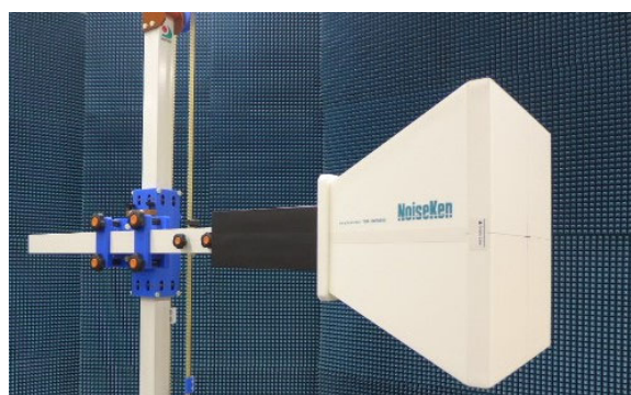
TEMホーン(製品), アンテナ長 60 cm
